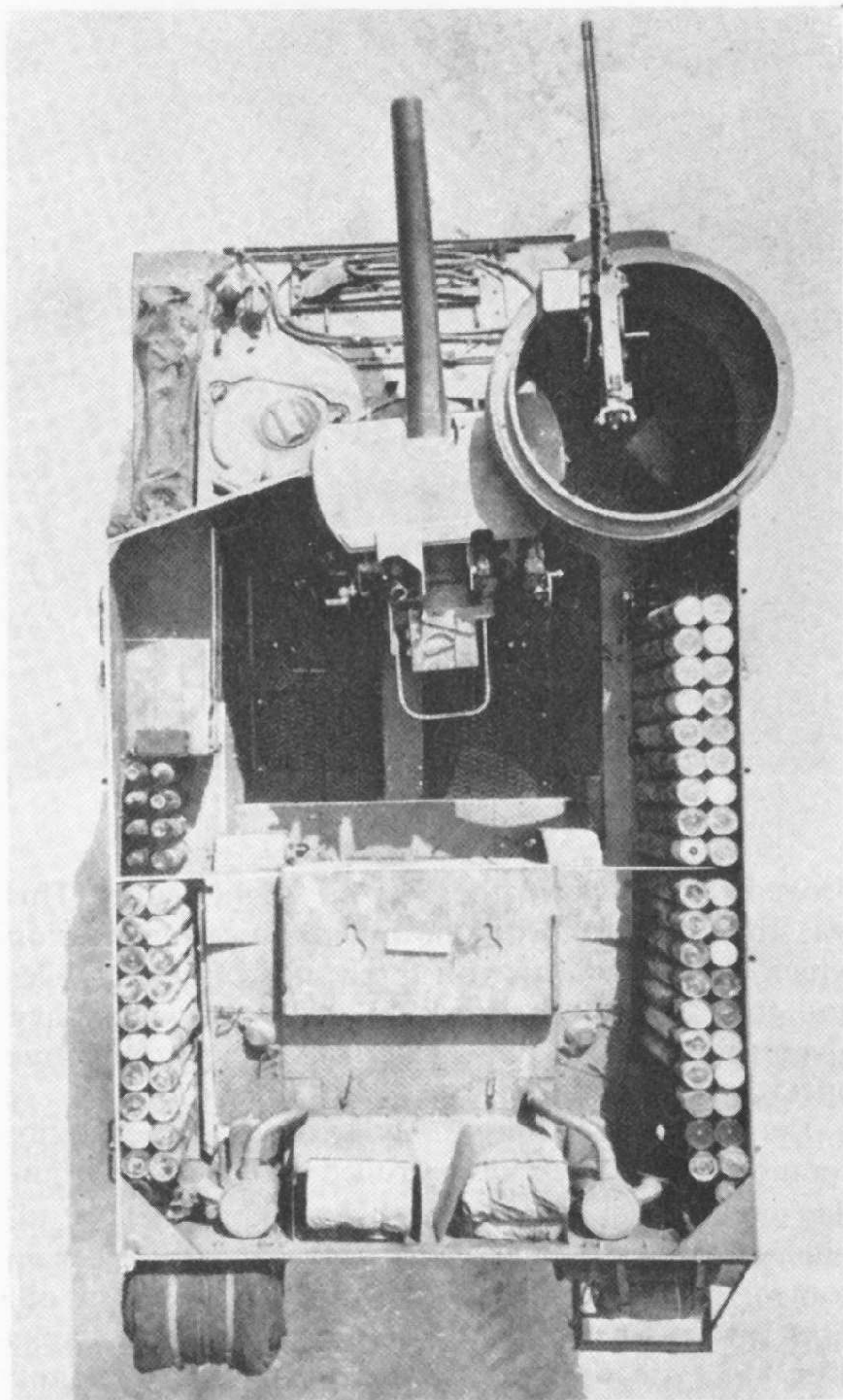
M.37 (T.76) 105 mm. HMC.
